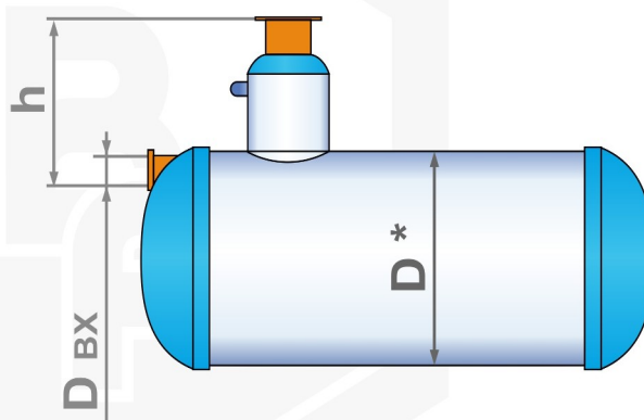
ГОРИЗОНТАЛЬНАЯ УСТАНОВКА
